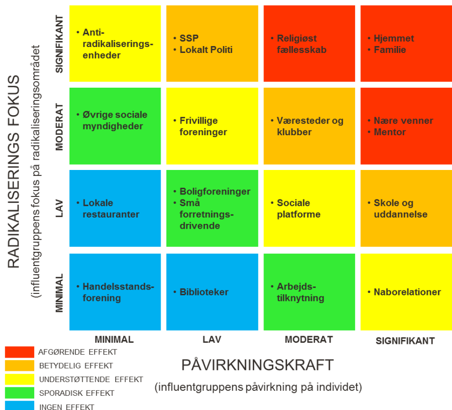
Figur 3: Resiliensmodel
